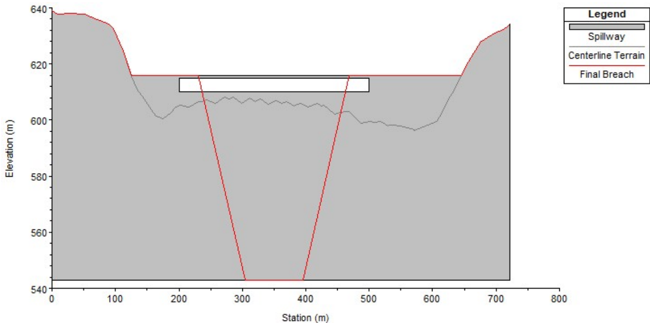
FIGURA 4.9 SEÇÃO MODELADA DA UHE DRJ E BRECHA FINAL DA RUPTURA: CENÁRIO TR 10,000 ANOS E ROMPIMENTO DA UHE SCL
