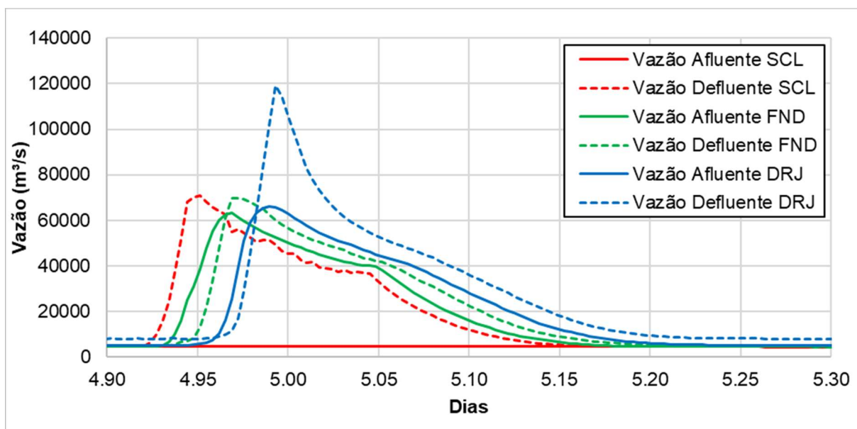
FIGURA 4.18 HIDROGRAMAS AFLUENTES E DEFLUENTES AOS RESERVATÓRIOS (DETALHE DO MOMENTO DA RUPTURA): CENÁRIO TR 10,000 ANOS E ROMPIMENTO DA UHE SCL
