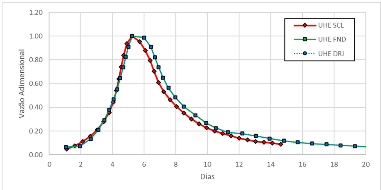
FIGURA 3.2 HIDROGRAMAS ADIMENSIONAIS DAS USINAS
