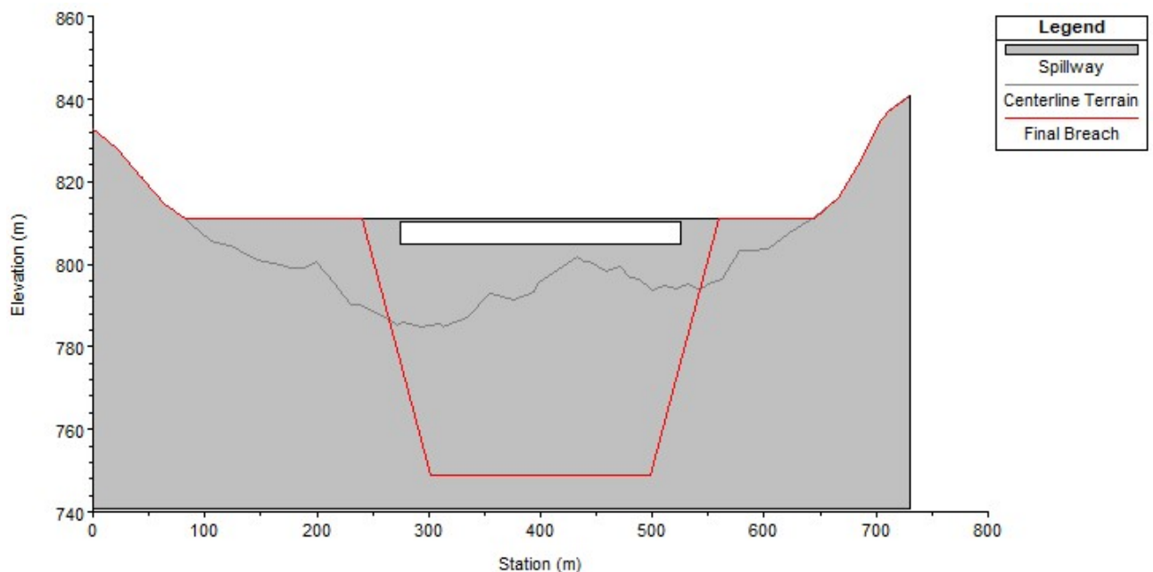
FIGURA 4.7 SEÇÃO MODELADA DA UHE SCL E BRECHA FINAL DA RUPTURA: CENÁRIO TR 10,000 ANOS E ROMPIMENTO DA UHE SCL
