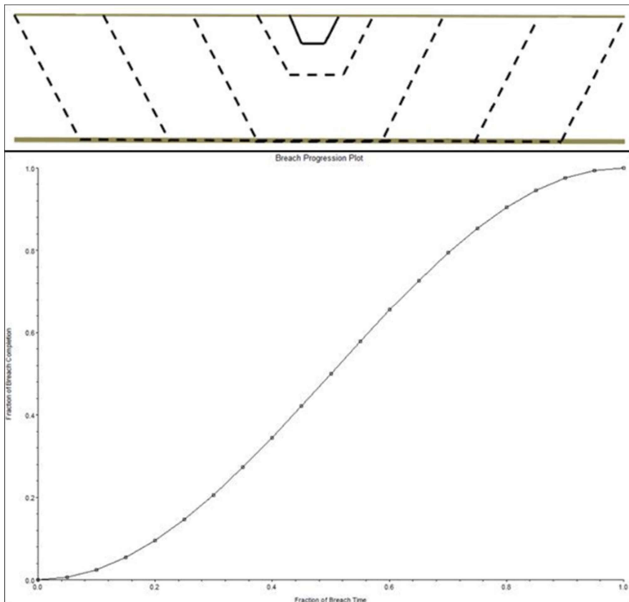
FIGURA 4.10 PROGRESSÃO DA BRECHA NO TEMPO
