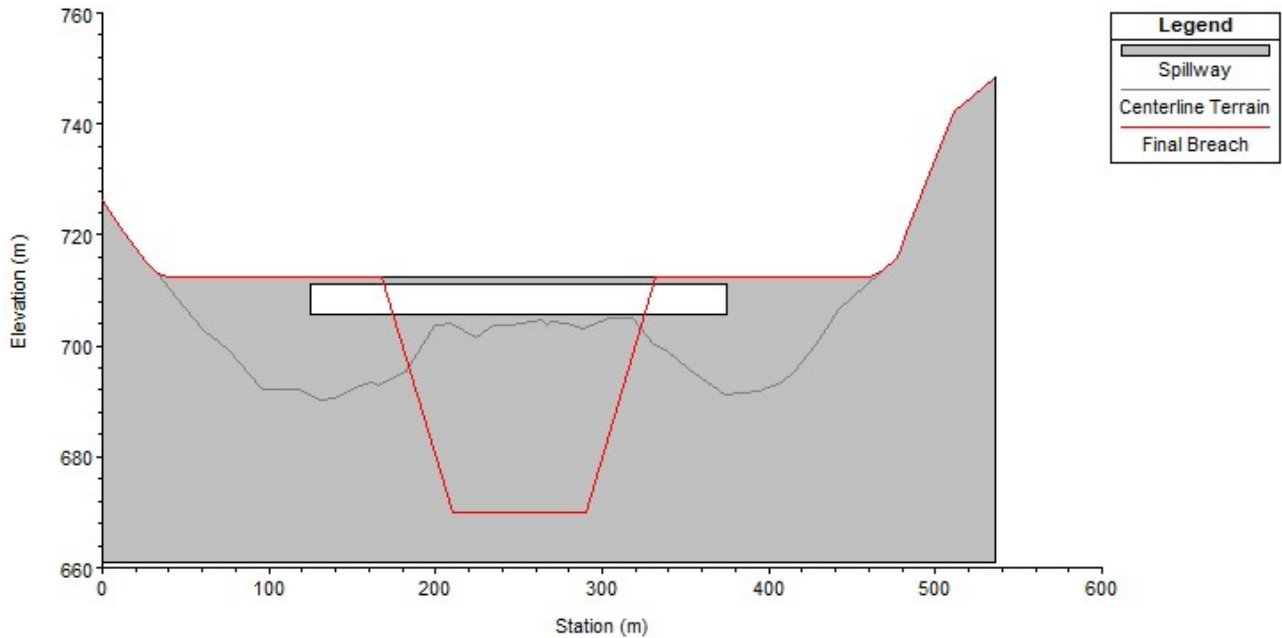
FIGURA 4.8 SEÇÃO MODELADA DA UHE FND E BRECHA FINAL DA RUPTURA: CENÁRIO TR 10,000 ANOS E ROMPIMENTO DA UHE SCL
