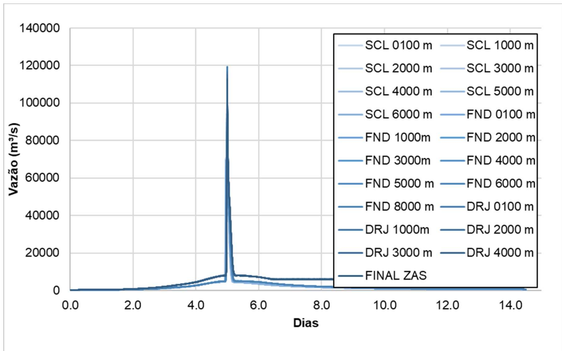
FIGURA 4.16 HIDROGRAMAS AFLUENTES E DEFLUENTES AOS RESERVATÓRIOS: CENÁRIO TR 10,000 ANOS E ROMPIMENTO DA UHE SCL
