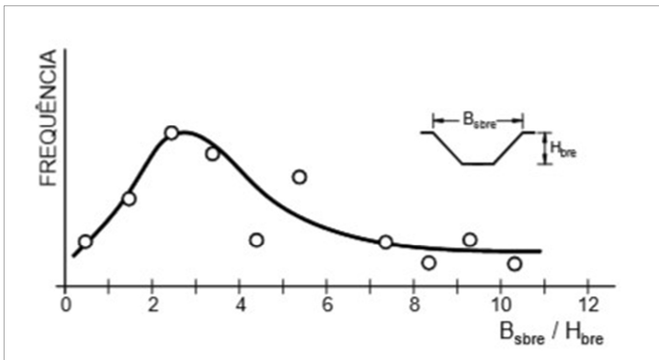
FIGURA 4.4 Curva de frequência B_{sbre}/H_{bre}
