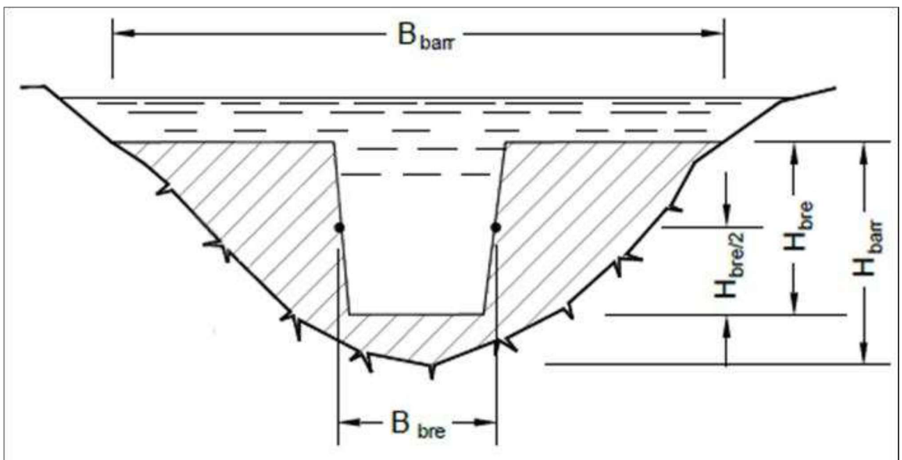
FIGURA 4.3 BRECHA DE RUPTURA PARA BARRAGENS
