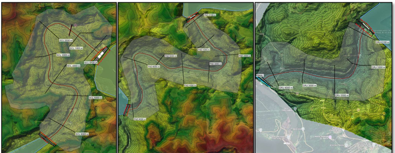
FIGURA 4.2 REGIÕES E MALHAS ADOTADAS PARA A MODELAGEM COMPUTACIONAL
